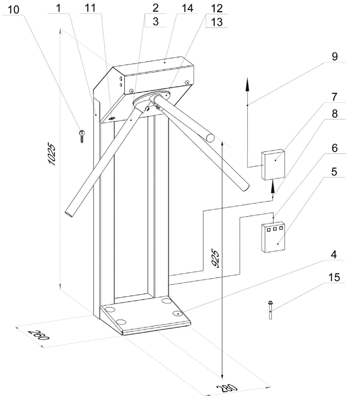
Рисунок 1 - Общий вид турникета
