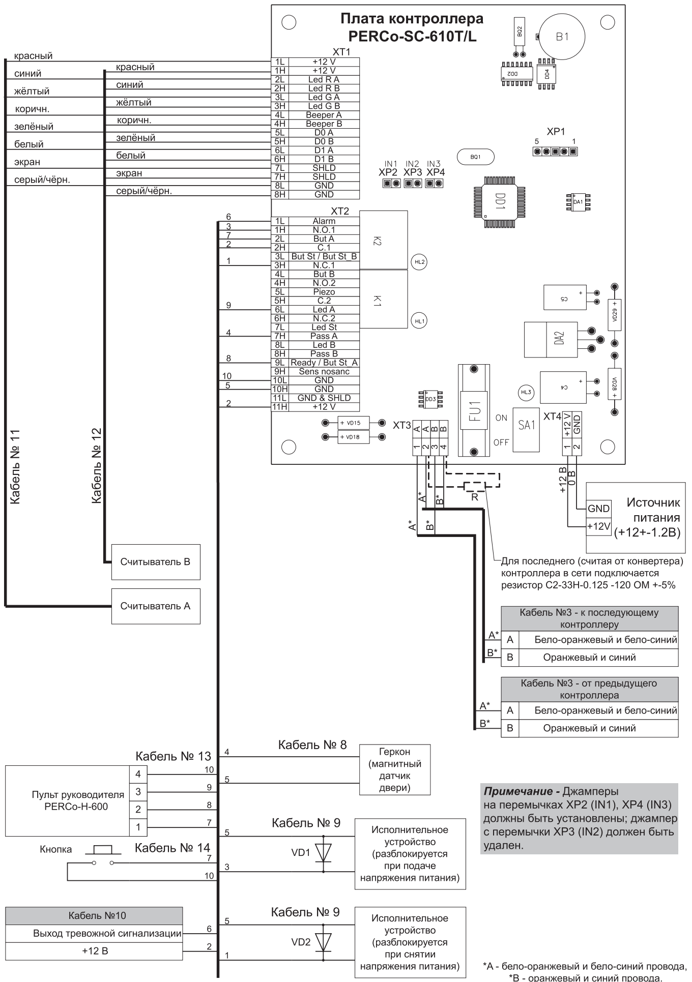
Схема 14- Схема монтажа контроллера PERCo-SC-610T/L (вариант "Замок" — оба считывателя привязаны к исполнительному устройству "А")
