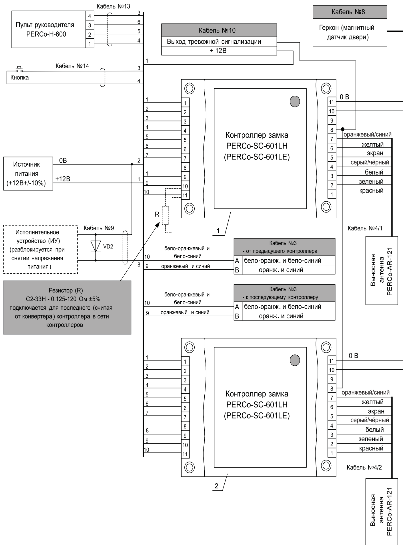
Схема 4г- Схема монтажа контроллеров замка PERCo-SC-601LH (LE) при организации входа и выхода в помещение по бесконтактным картам доступа
