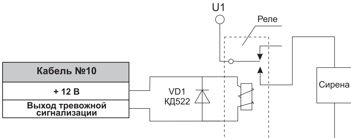
Рисунок 3 - Пример гальванической развязки цепи
