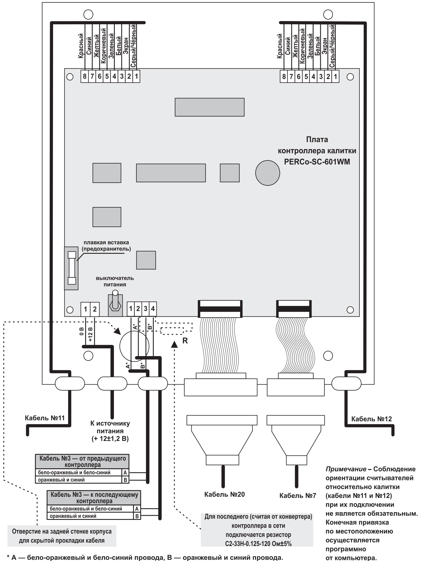
Схема 12- Схема монтажа контроллера калитки электромеханической PERCo-SC-601WM
