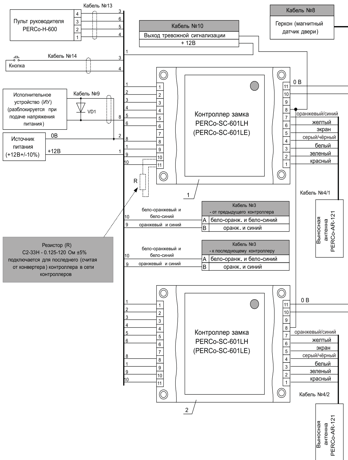
Схема 4в- Схема монтажа контроллеров замка PERCo-SC-601LH (LE) при организации входа и выхода в помещение по бесконтактным картам доступа
