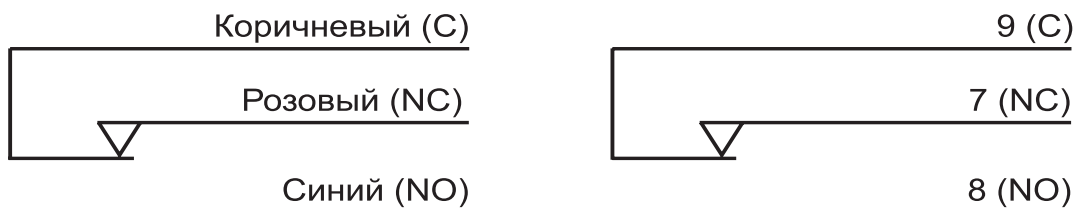
Рисунок 4 - Выходное реле замковых контроллеров PERCo-SC600LH (LE) с указанием цвета проводов. Выходное реле замковых контроллеров PERCo-SC601LH (LE) с указанием номеров контактов
