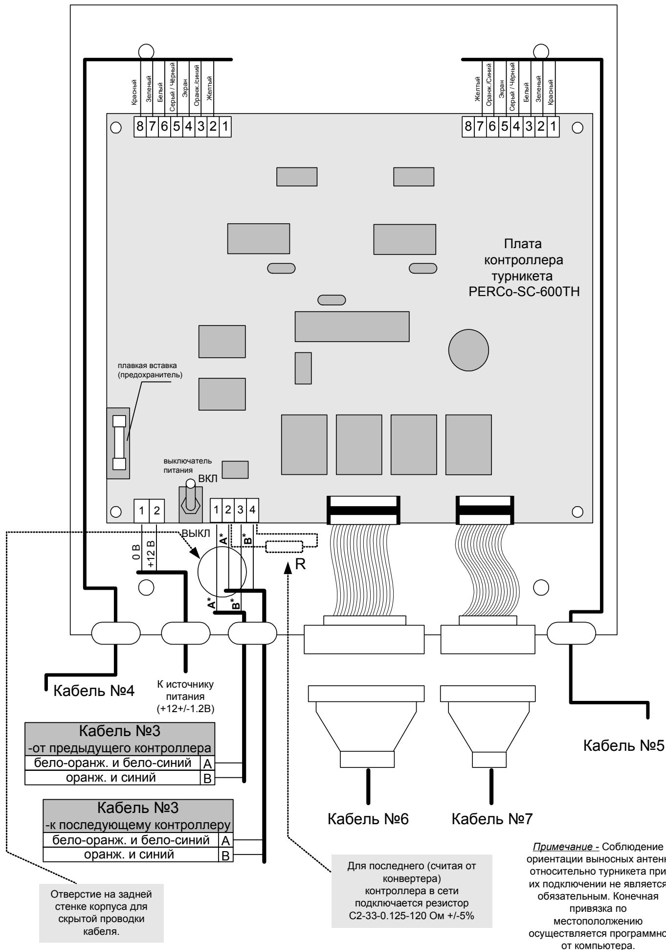
Схема 7- Схема монтажа контроллера турникета PERCo-SC-600TH
