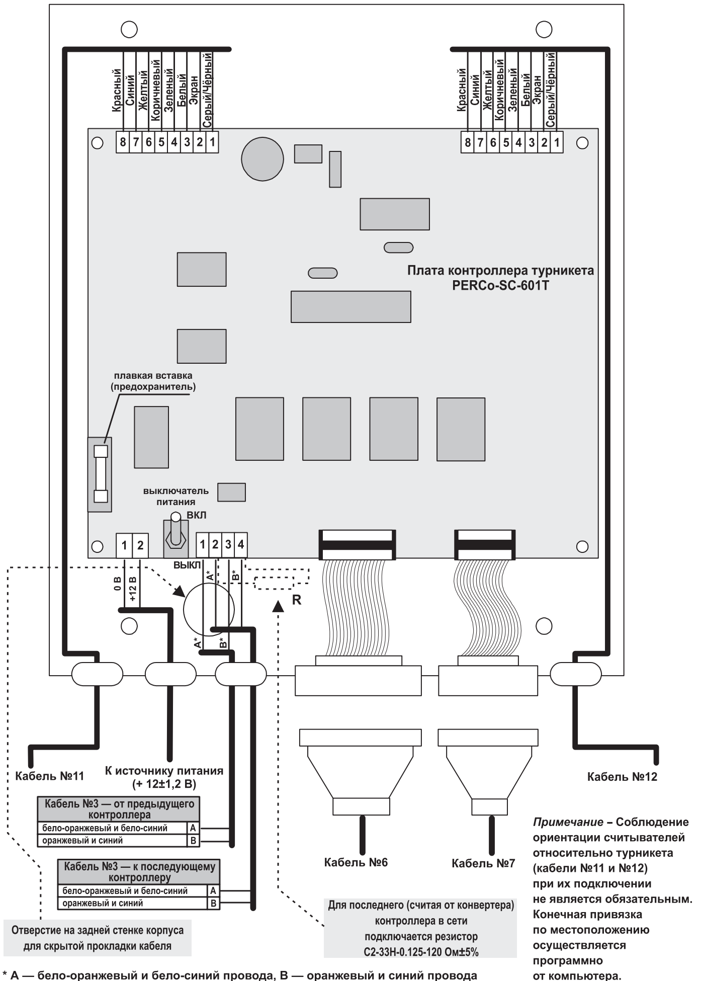
Схема 8- Схема монтажа контроллера турникета PERCo-SC-601T
