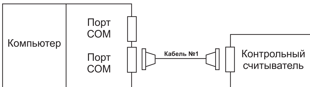
Рисунок 2 - Схема установки контрольного считывателя
