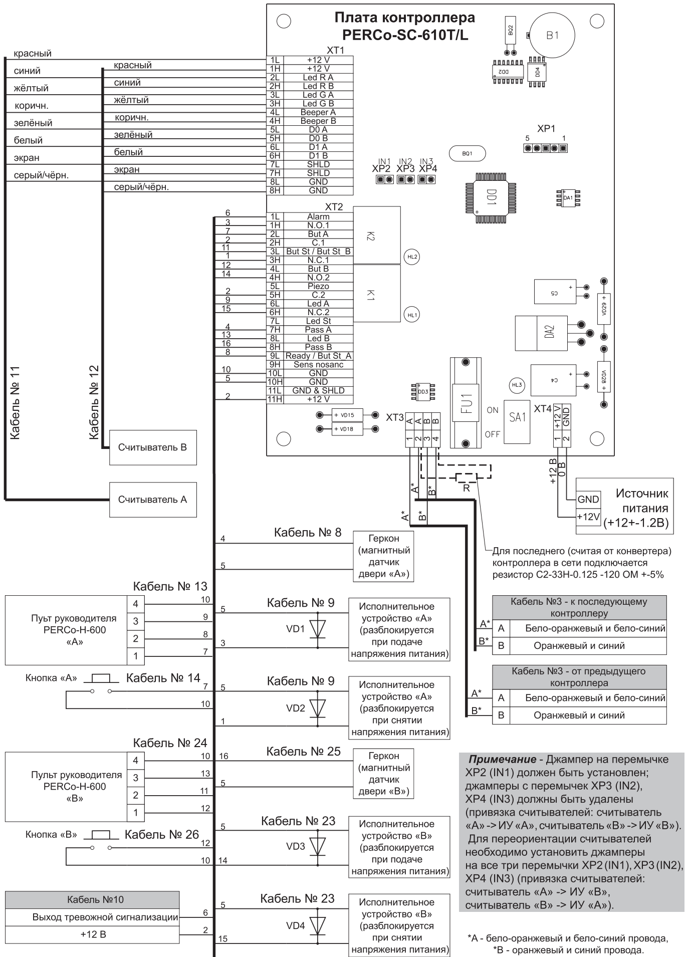
Схема 16- Схема монтажа контроллера PERCo-SC-610T/L (вариант "Два замка")
