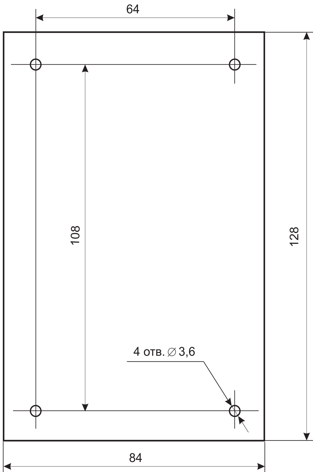
Рисунок 1- Разметка отверстий для установки конвертера интерфейса PERCo-IC-600, контроллеров замка PERCo-SC-600LH (LE), PERCo-SC-601LH (LE) и выносной антенны PERCo-AR-121
