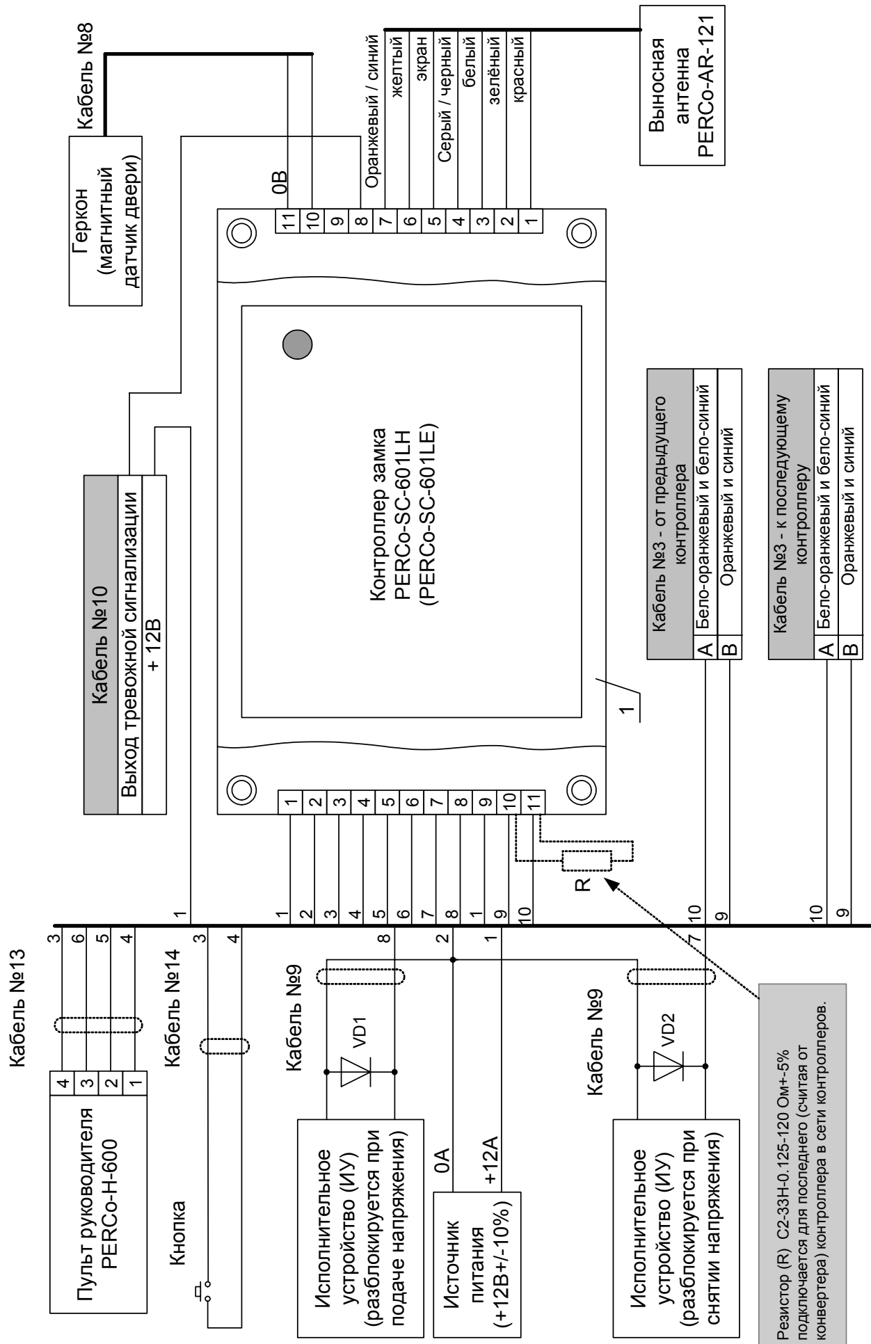
Схема 3- Схема монтажа контроллеров замка PERCo-SC-601LH (LE)
