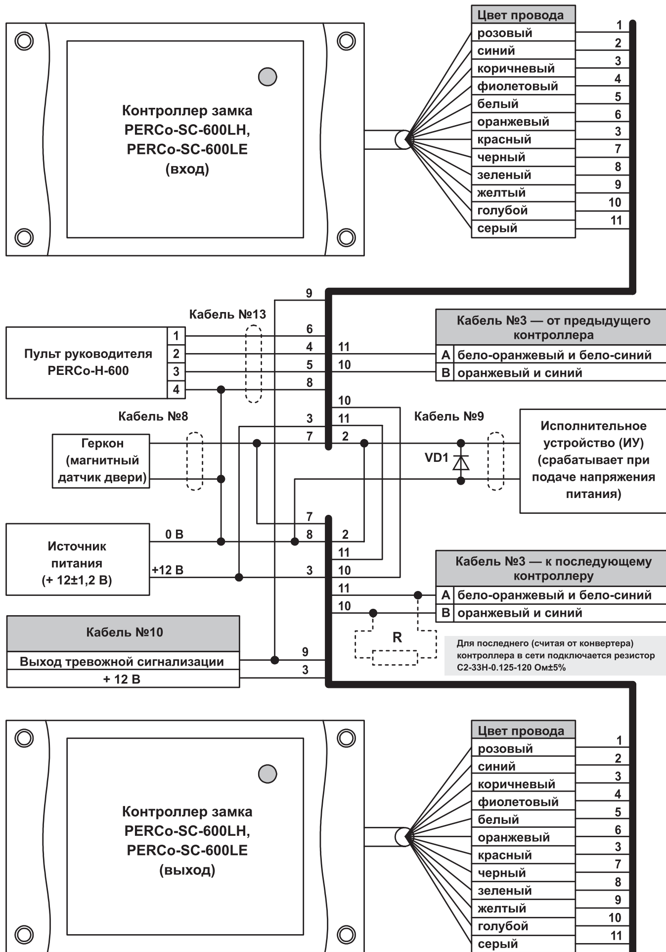
Схема 4а- Схема монтажа контроллеров замка PERCo-SC-600LH (LE) при организации входа и выхода в помещение по бесконтактным картам доступа.
