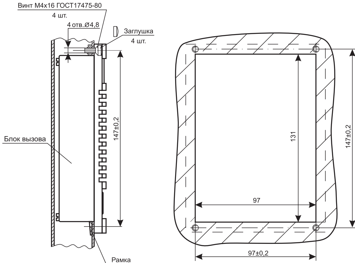
Рисунок 5 - Установка контроллера PERCo-SC-600PDP (PERCo-SC-600PDPV) на металлическую дверь
