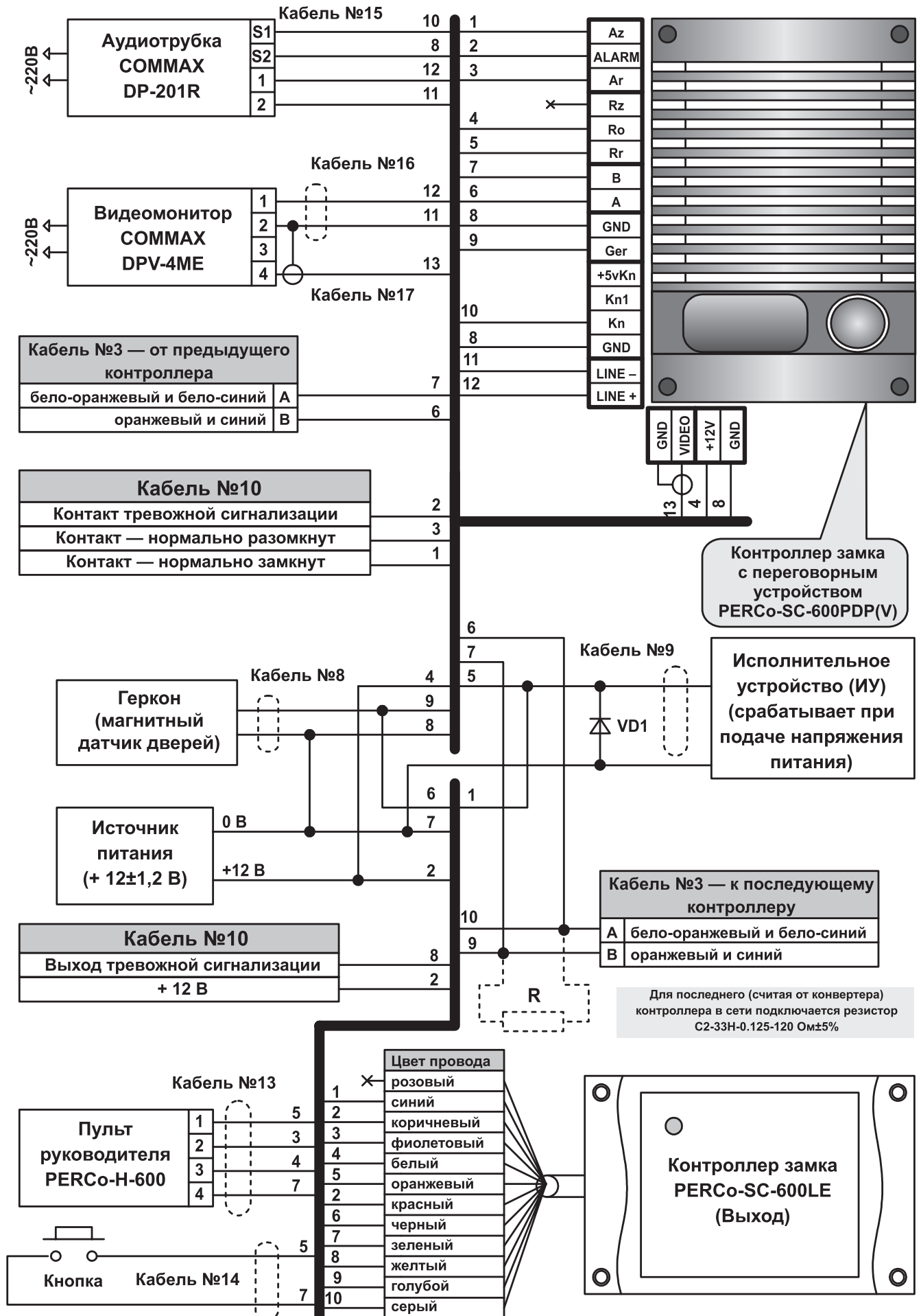
Схема 6- Схема подключения контроллера замка PERCo-SC-600LE и контроллера замка с переговорным устройством PERCo-SC-600PDP(V)
