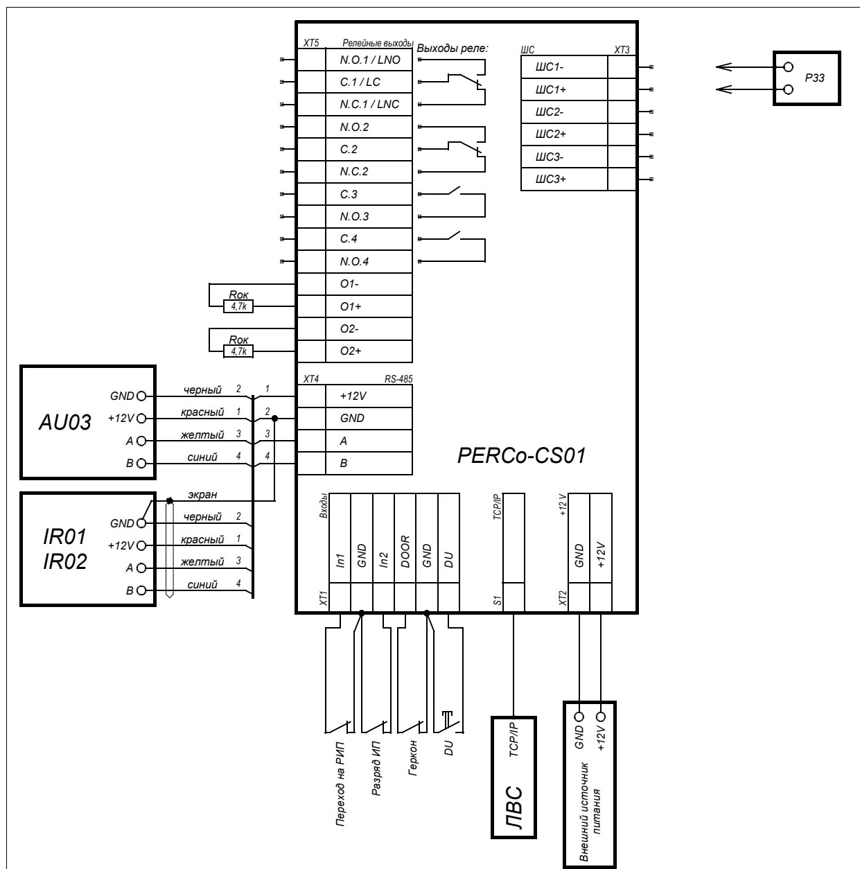
Рисунок Е.2 – Схема подключения ППКОП – Контроллера безопасности объекта PERCo-CS01 при проверке технического состояния
