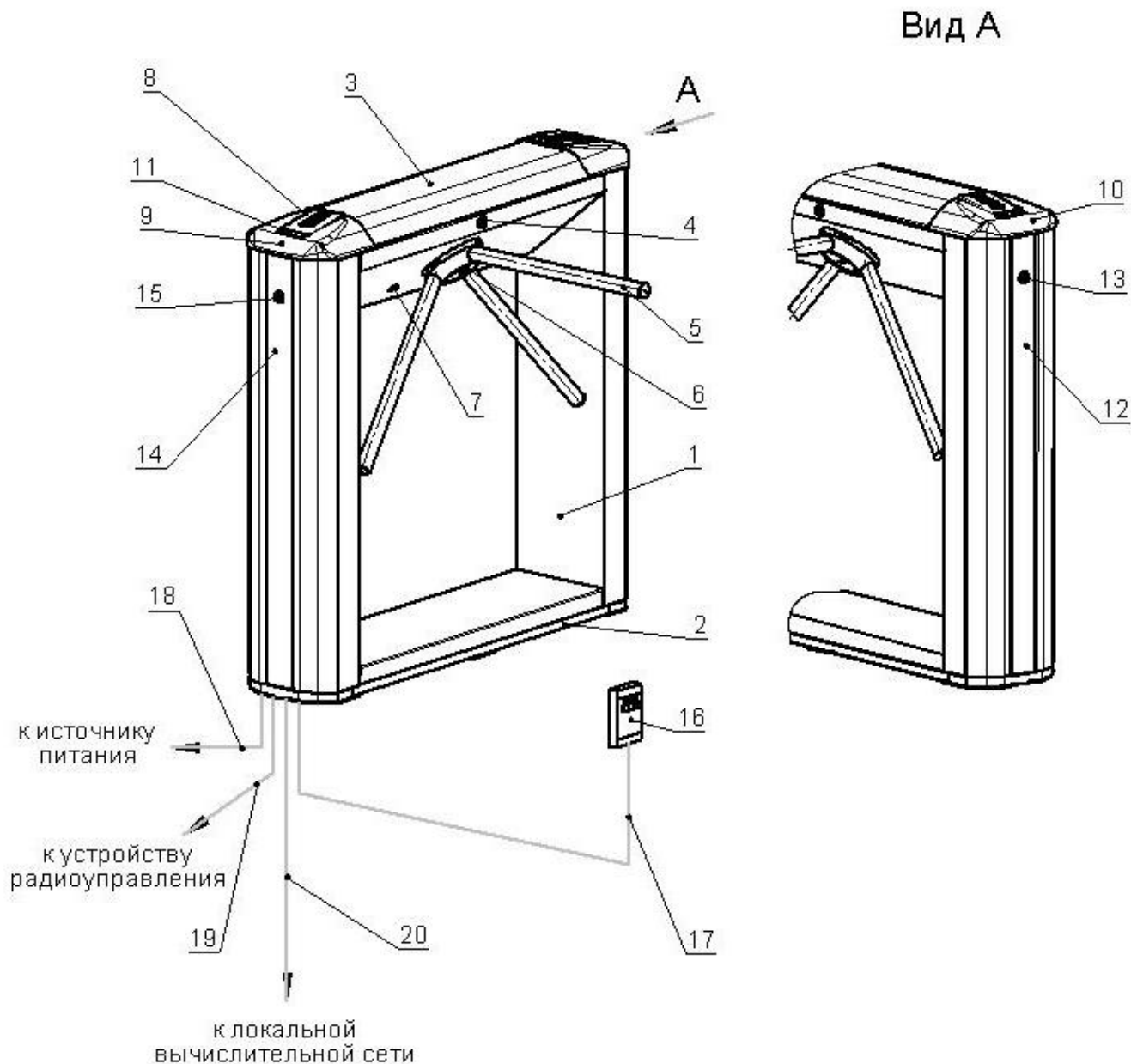
Рисунок 1 – Устройство КТ05.3
