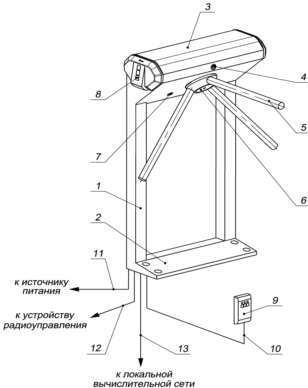
Рисунок 1 – Устройство ЭП:
