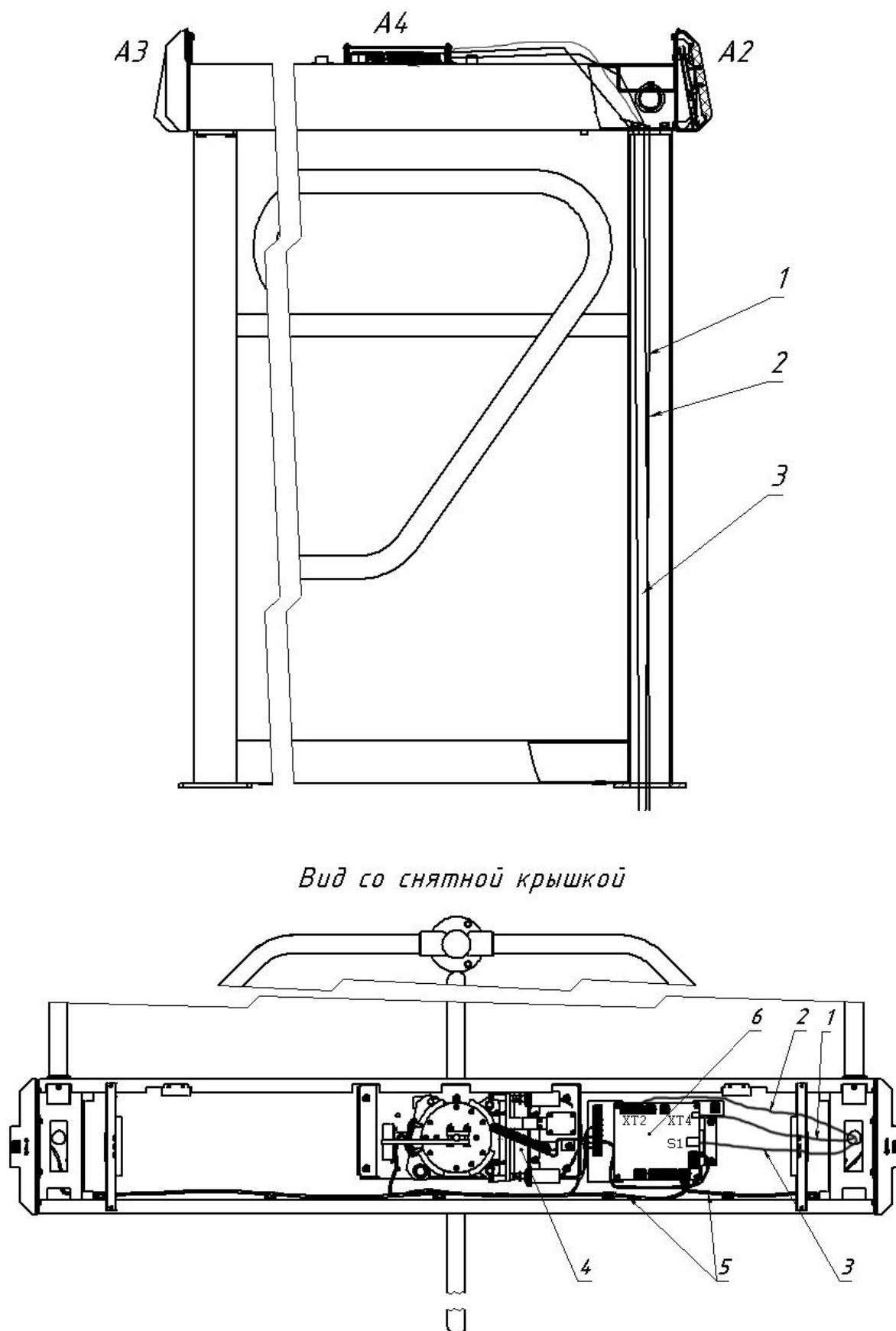
Рисунок 7 – Схема прокладки кабелей в стойке ЭП:
