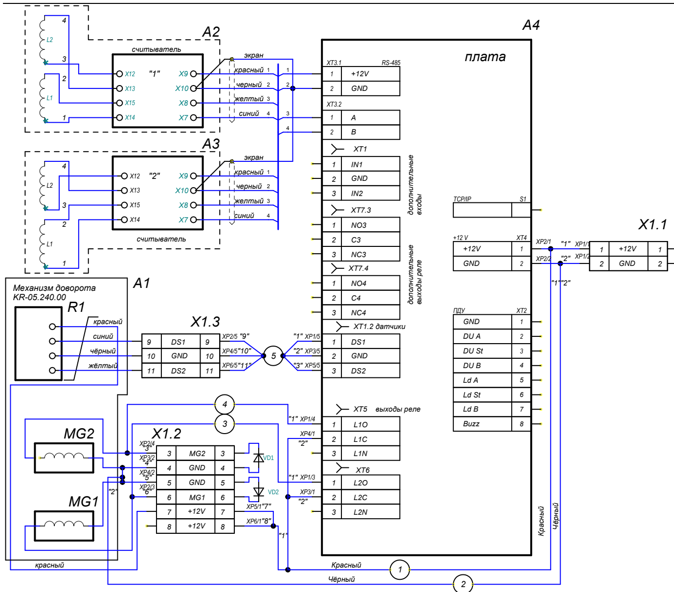
Рисунок А.2 – Схема внутренних соединений ЭП*
